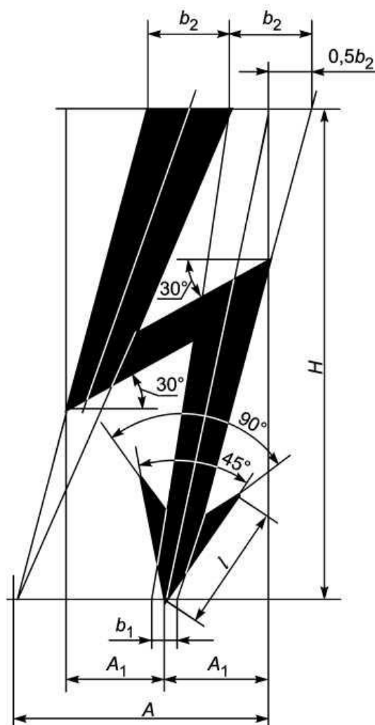
Рисунок Н.1 — Графический символ электрического напряжения
